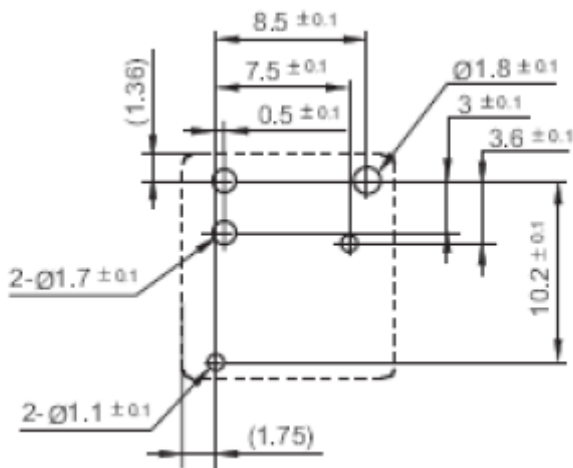
PCB 安装图
